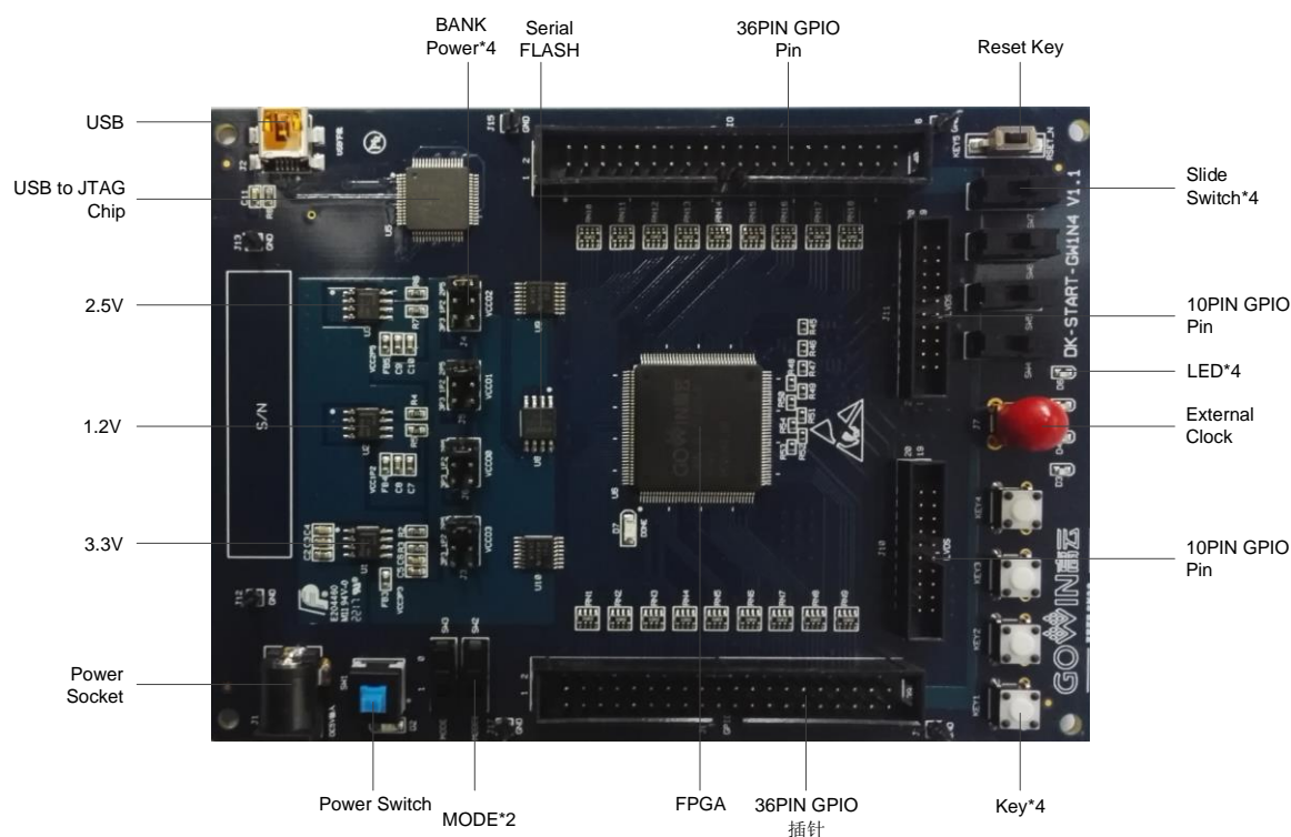
図1 PCB コンポーネント
