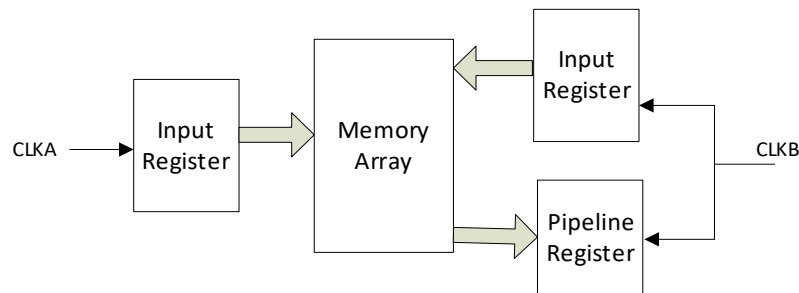
シングル・ポート・クロックモード
