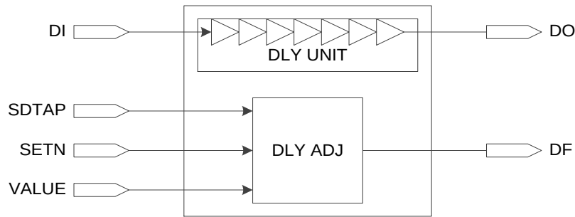
図 2-13 IODELAY の説明図
