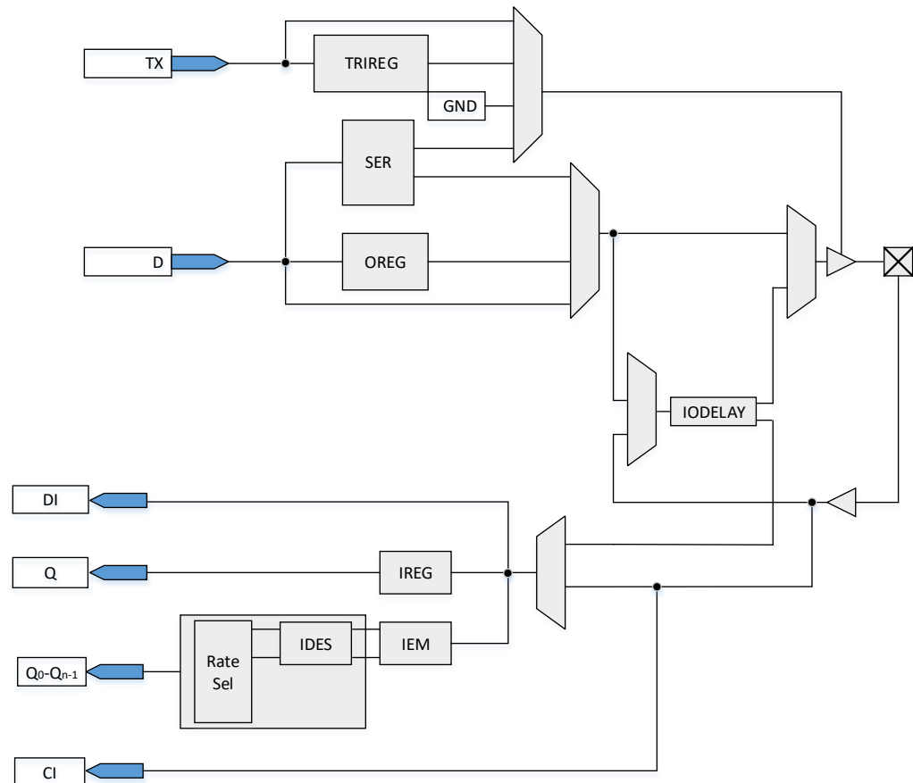
図 2-12 I/O ロジックの入力と出力の説明図
