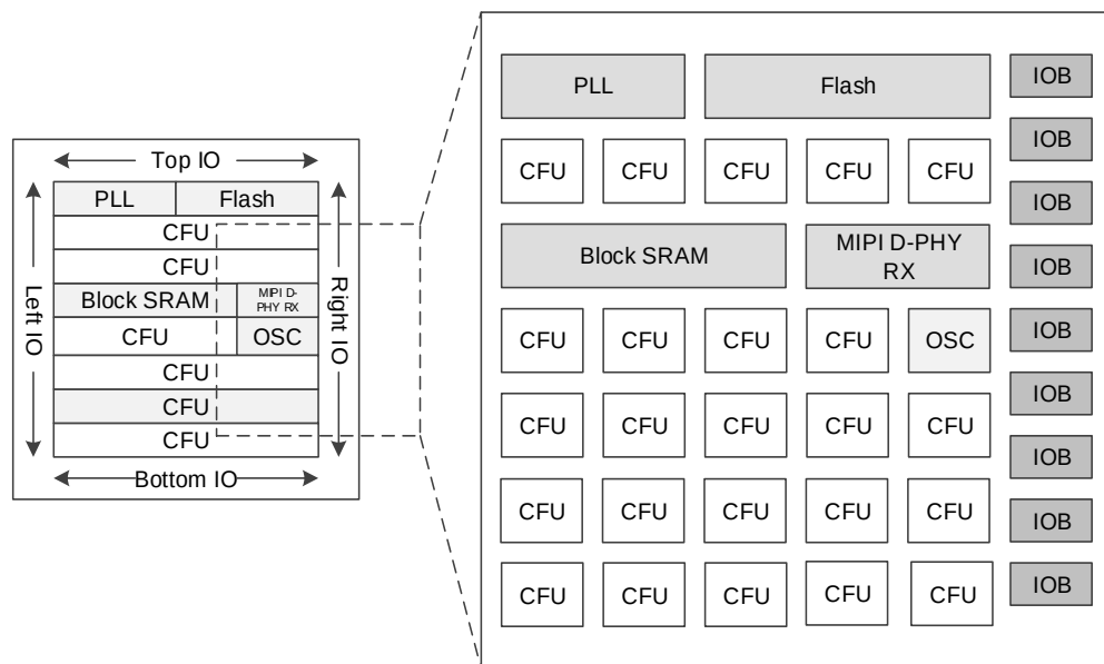
図 2-4 GW1N シリーズ FPGA デバイス(GW1N-2)の構造
