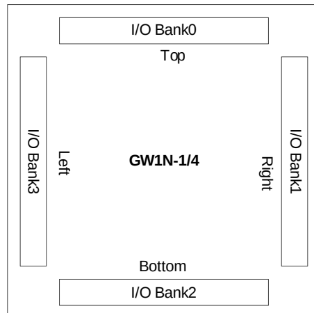
図 2-7 GW1N-1/4 の I/O Bank の配置図
