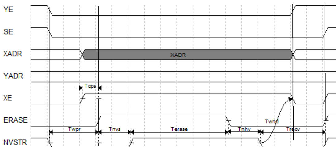
図 3-7 User Flash の消去タイミング
