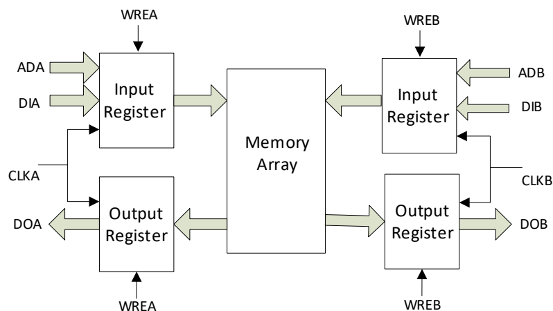
図 2-16 独立クロックモード
