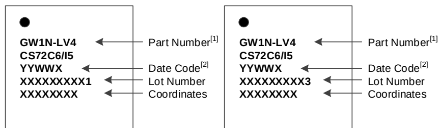
図 4-4 デバイスのパッケージのマーク例(GW1N-LV4CS72C6/I5)
