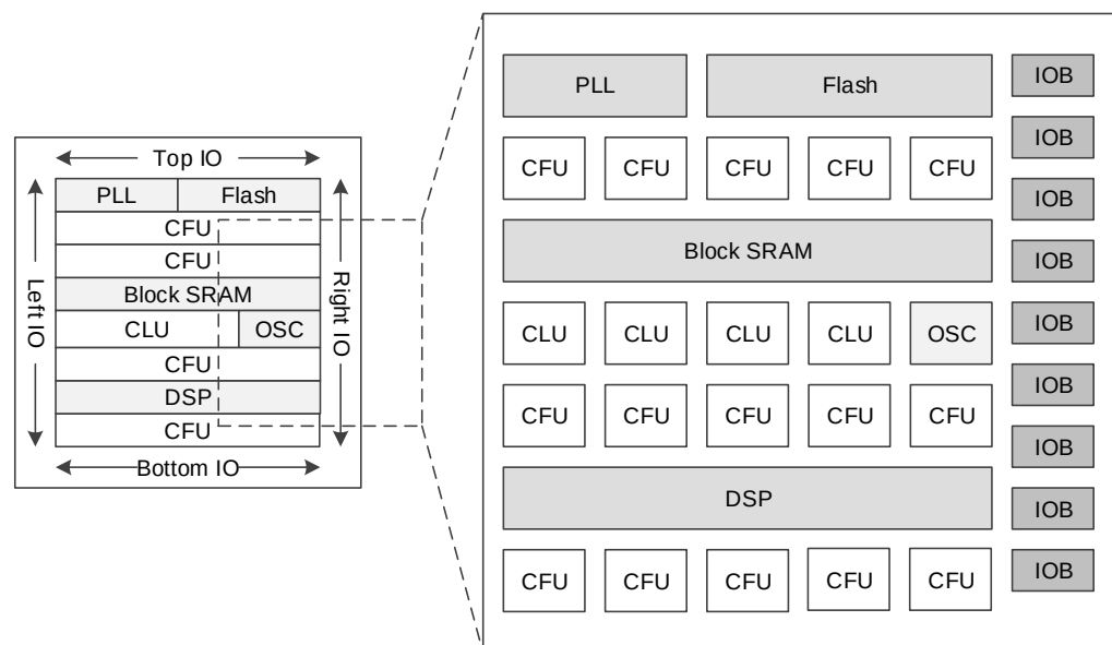
図 2-1 GW1N シリーズ FPGA デバイス(GW1N-9)の構造
