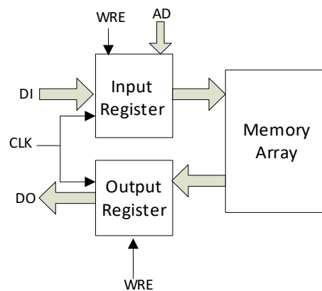
図 2-18 シングル・ポート・クロックモード
