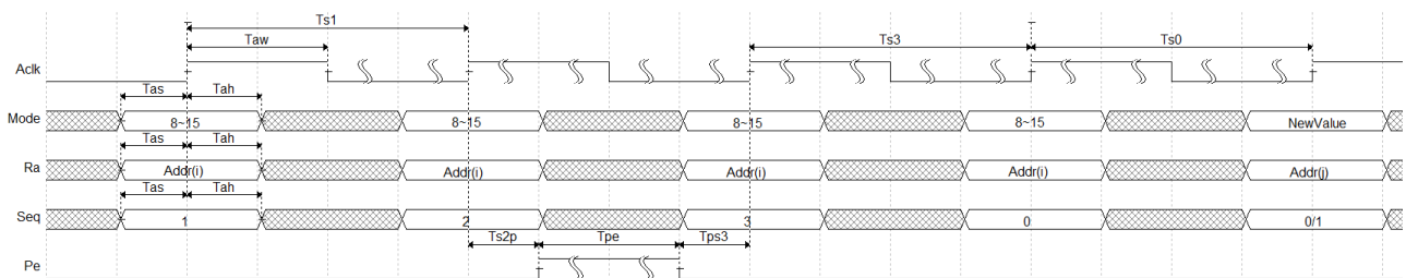
図 3-4 High レベルサイクル
