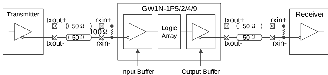
図 2-11 True LVDS 設計のブロック図
