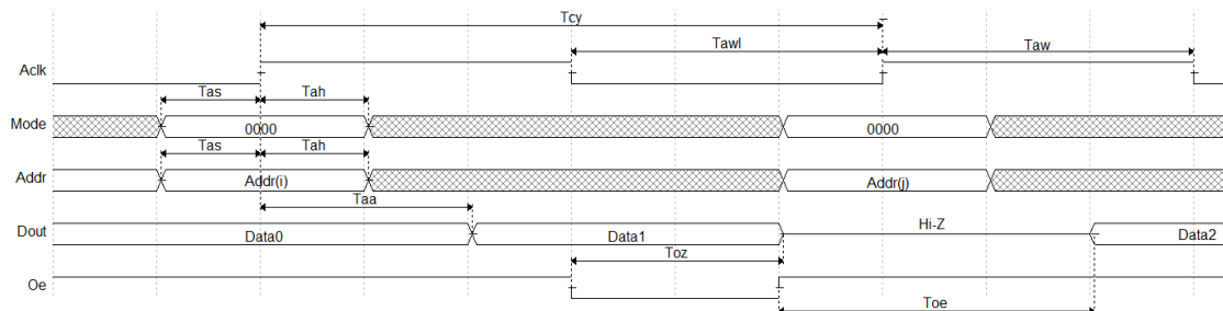
図 3-1 読み出しモード
