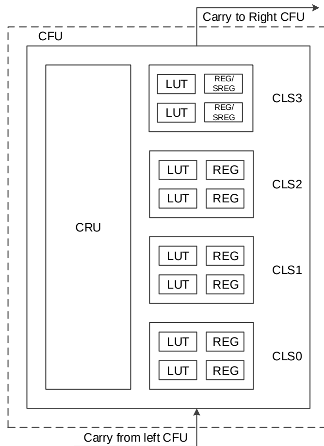
図 2-5 CFU 構造の説明図
