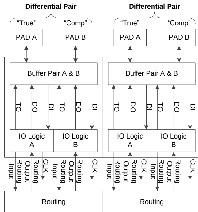
図 2-6 IOB 構造の説明図
