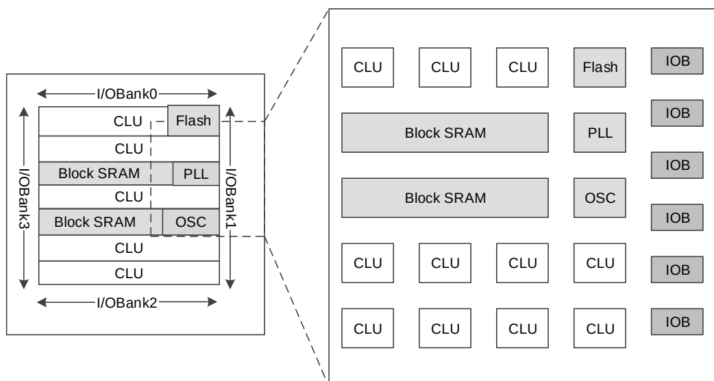
図 2-3 GW1N シリーズ FPGA デバイス(GW1N-1)の構造
