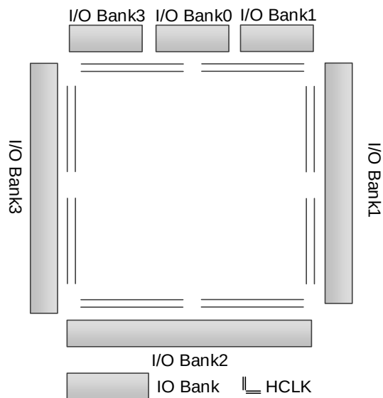
図 2-22 GW1N-9 HCLK の説明図
