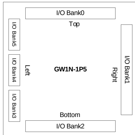
図 2-8 GW1N-1P5 の I/O Bank の配置図
