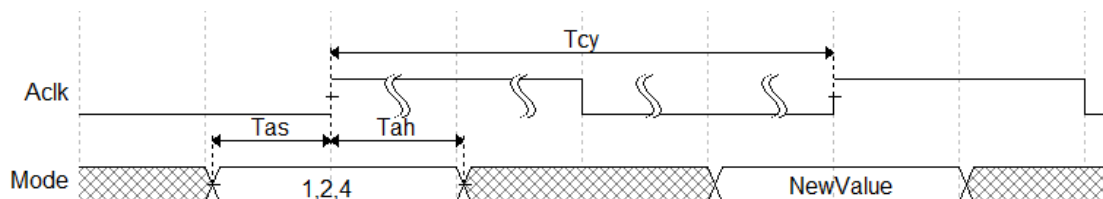
図 3-3 ページラッチ・クリア・モード
