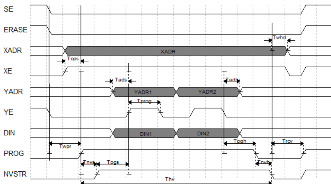
図 3-6 User Flash のプログラミングタイミング
