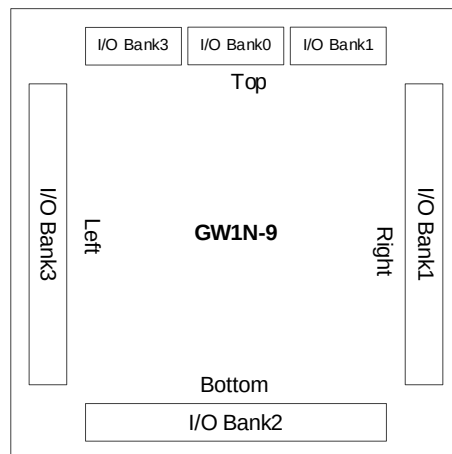
図 2-10 GW1N-9 の I/O Bank の配置図
