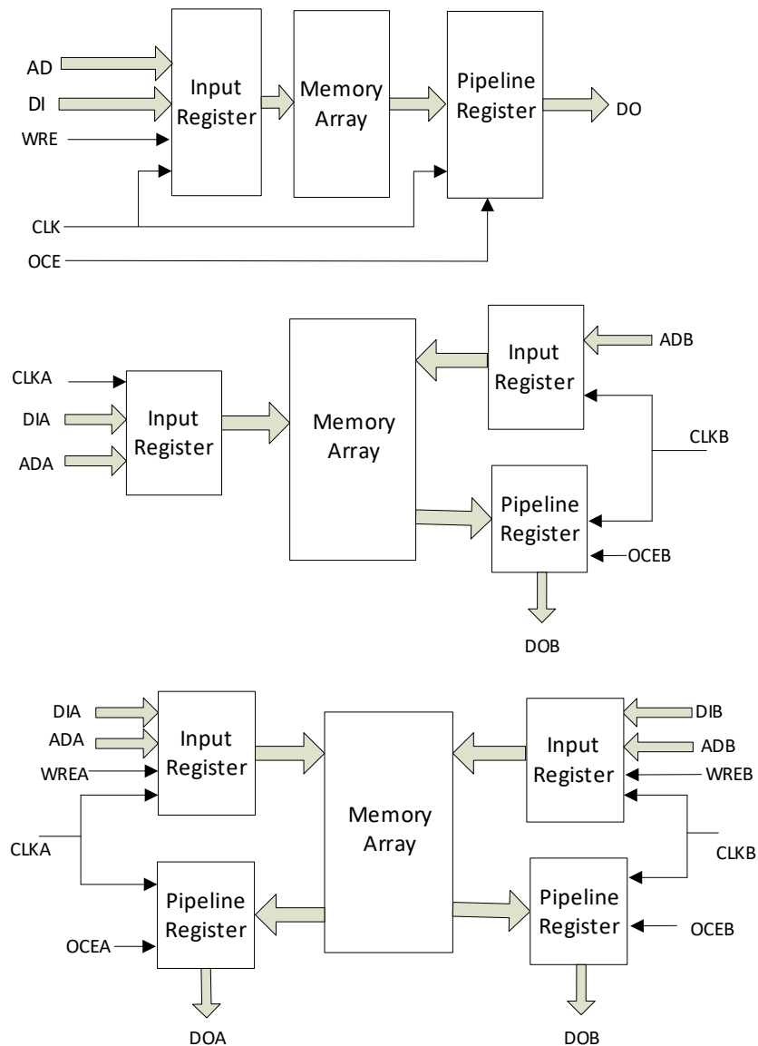
図 2-15 シングル・ポート、セミ・デュアル・ポート、及びデュアル・ポート・モードにおけるパイプラインモード
