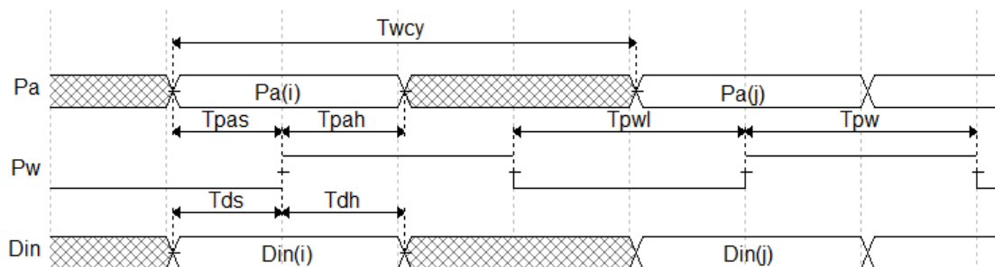
図 3-2 ページラッチ書き込みモード
