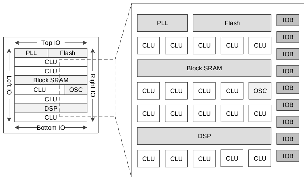
図 2-3 GW1N シリーズ FPGA デバイス(GW1N-1)の構造
