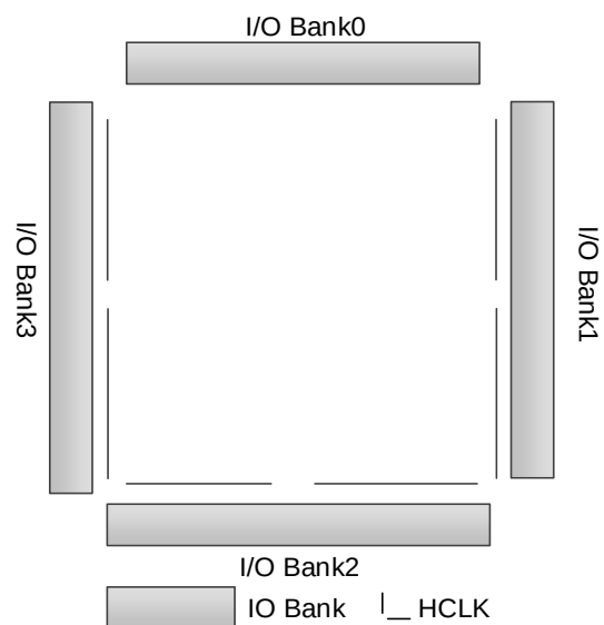
図 2-21 GW1N-4 HCLK の説明図
